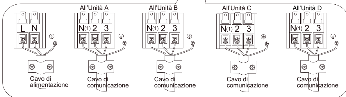
All'alimentazione elettrica
