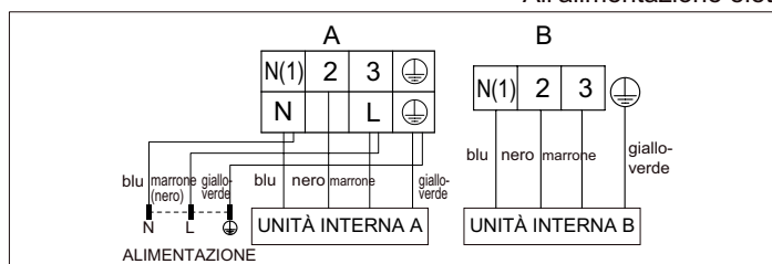
All'alimentazione elettrica
