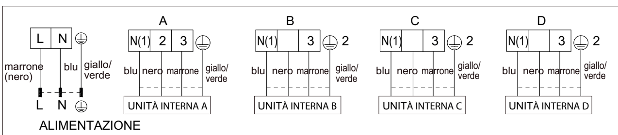
All'alimentazione elettrica
