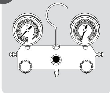
Esecuzione del vuoto dell'impianto
