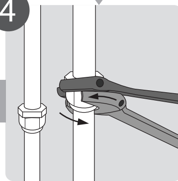
Collegamento delle tubazioni frigorifere
