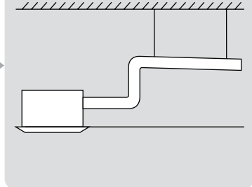
Installazione del tubo di scarico della condensa
