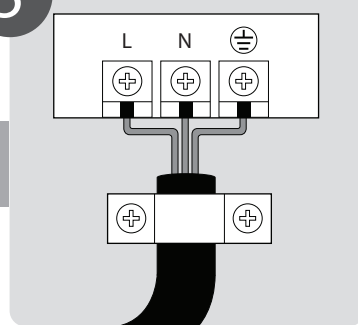
Collegamenti elettrici
